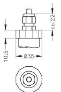
Кабельный ввод
