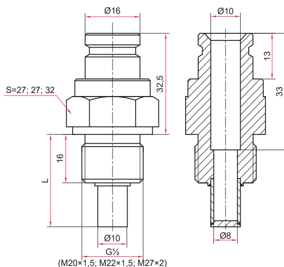
Гильза для термометров ТТ-В (РЧ Исп. 2 – угловые)
