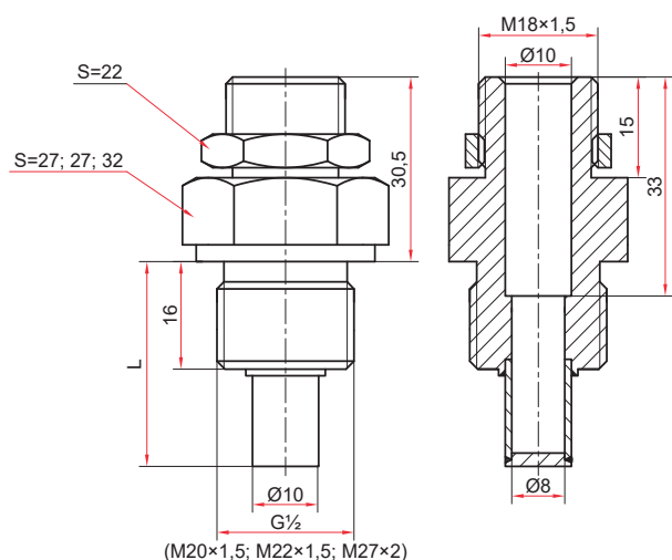
Гильза для термометров БТ серии 211
